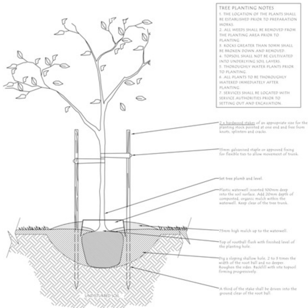
- TREE PLANTING DETAIL LO1 N.T.S.
